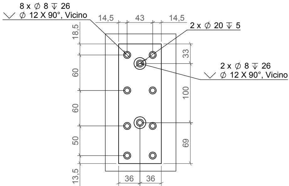
DETTAGLIO A
